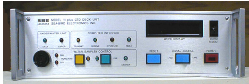
SBE 11 plus V2 Deck Unit
